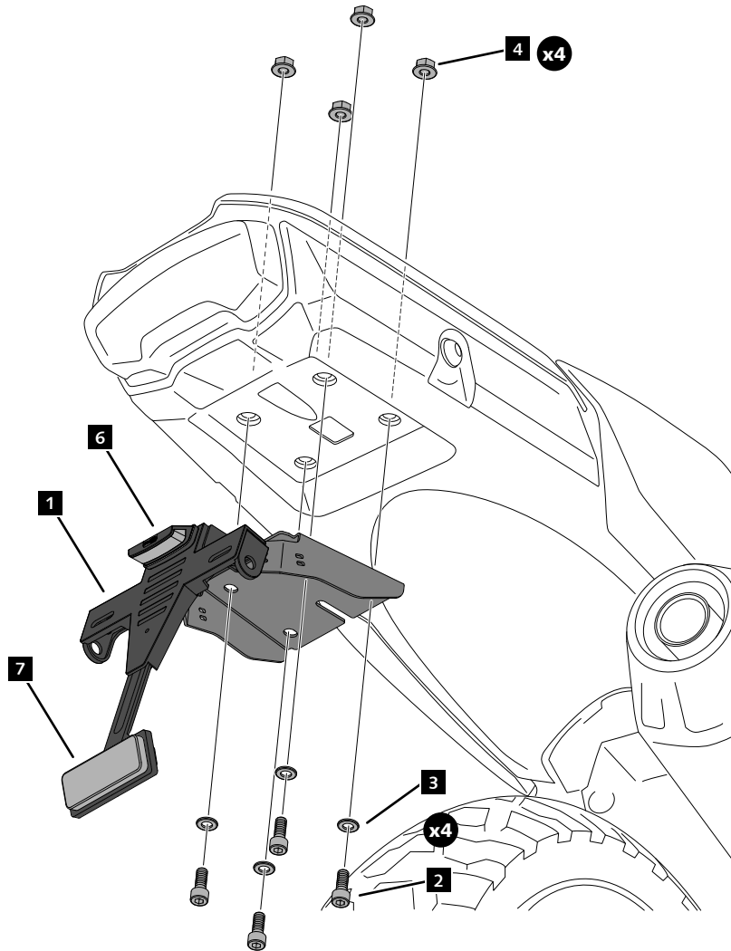
Fijación giro portamatrículas (2 OPCIONES A-B) Fixation license support rotation (2 OPTIONS A-B)
